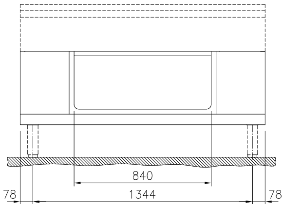
Front aanzicht
